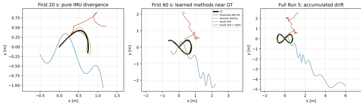
CF231 궤적 비교
