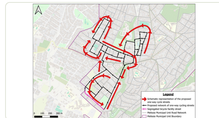
Le réseau de 5 km de rues cyclables — SUM D4.2, Fig. 34
