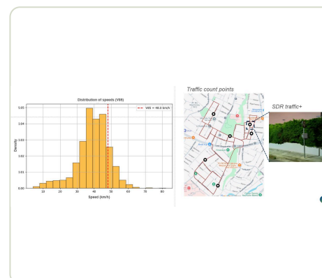
Vitesses mesurées avant travaux (V85 = 48 km/h) — SUM D4.2, Fig. 59
