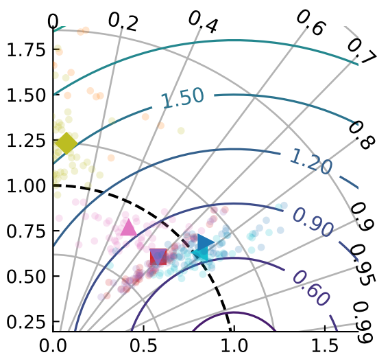
MIROC6
