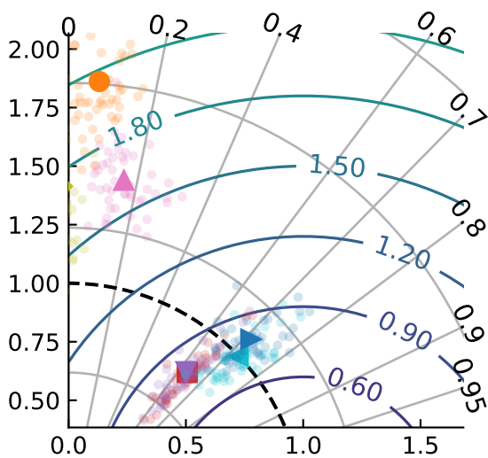
MIROC6
