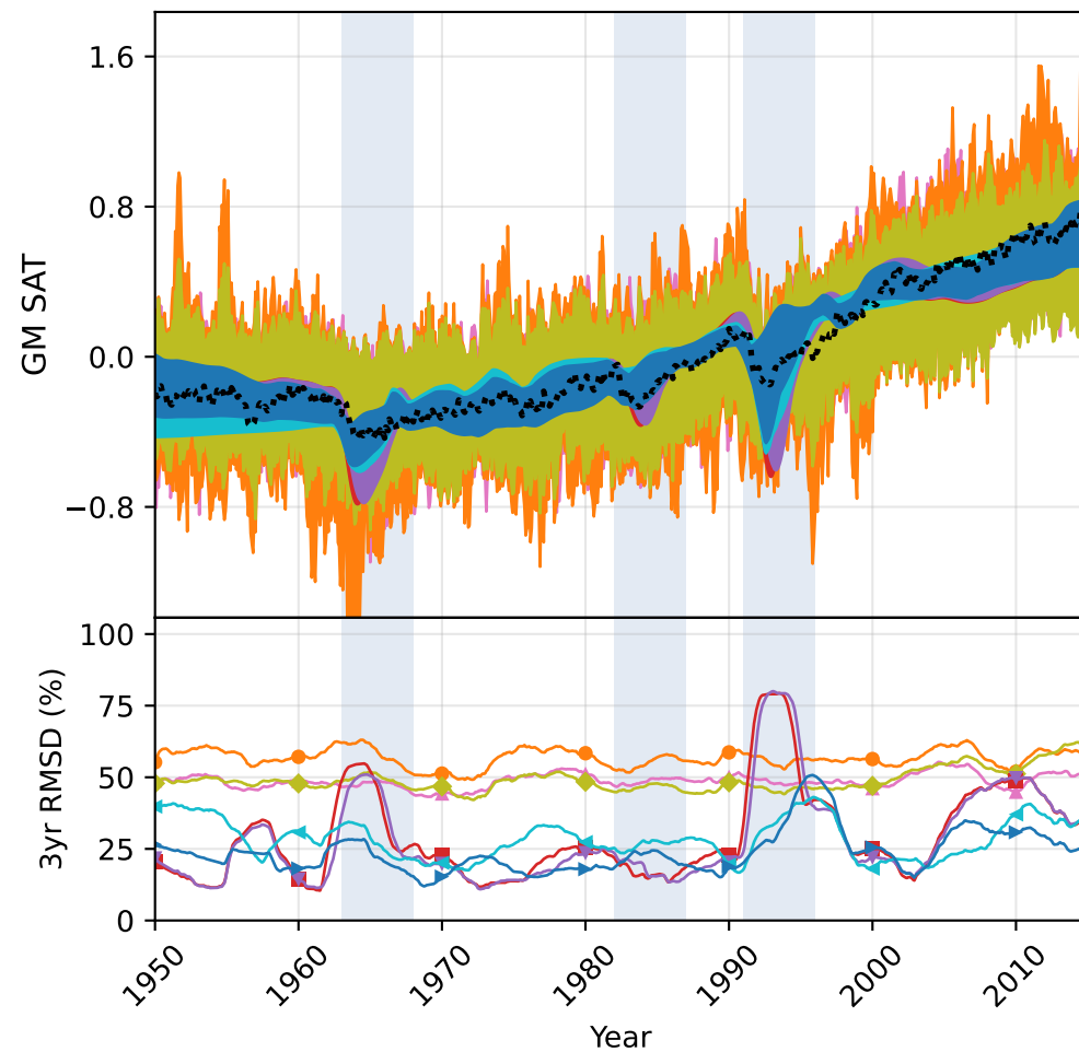
CESM2
