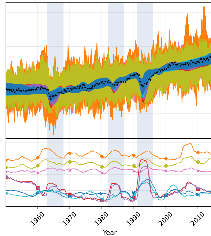
MPI-ESM
