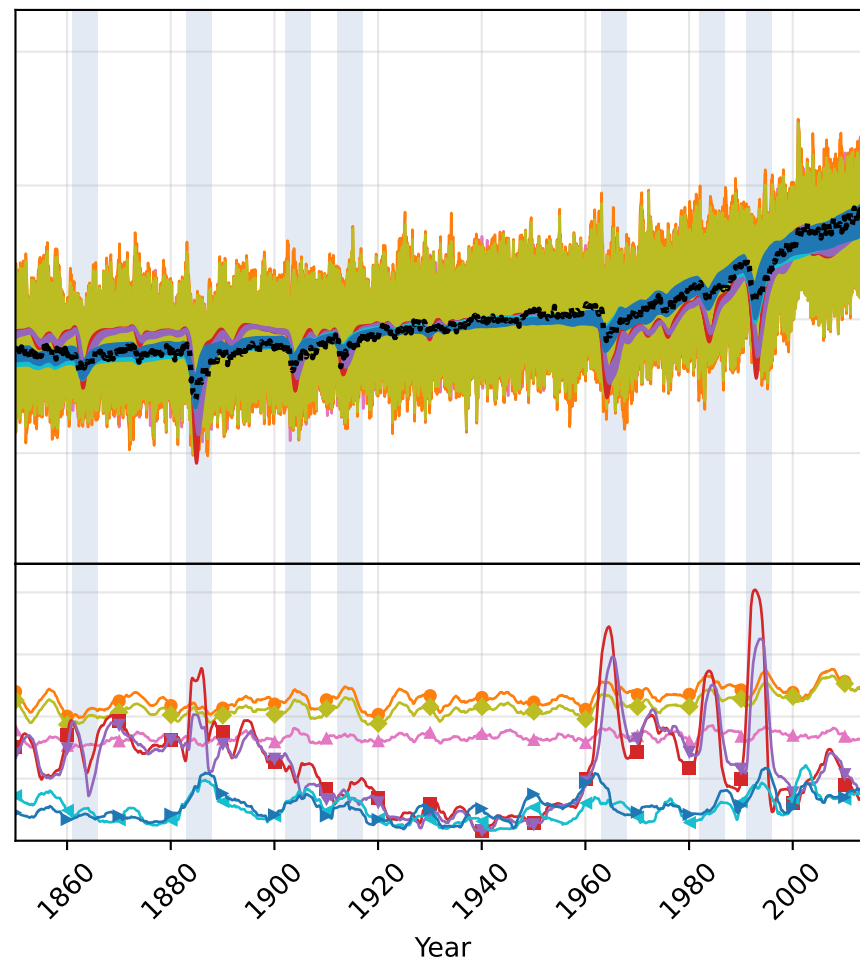
MPI-ESM
