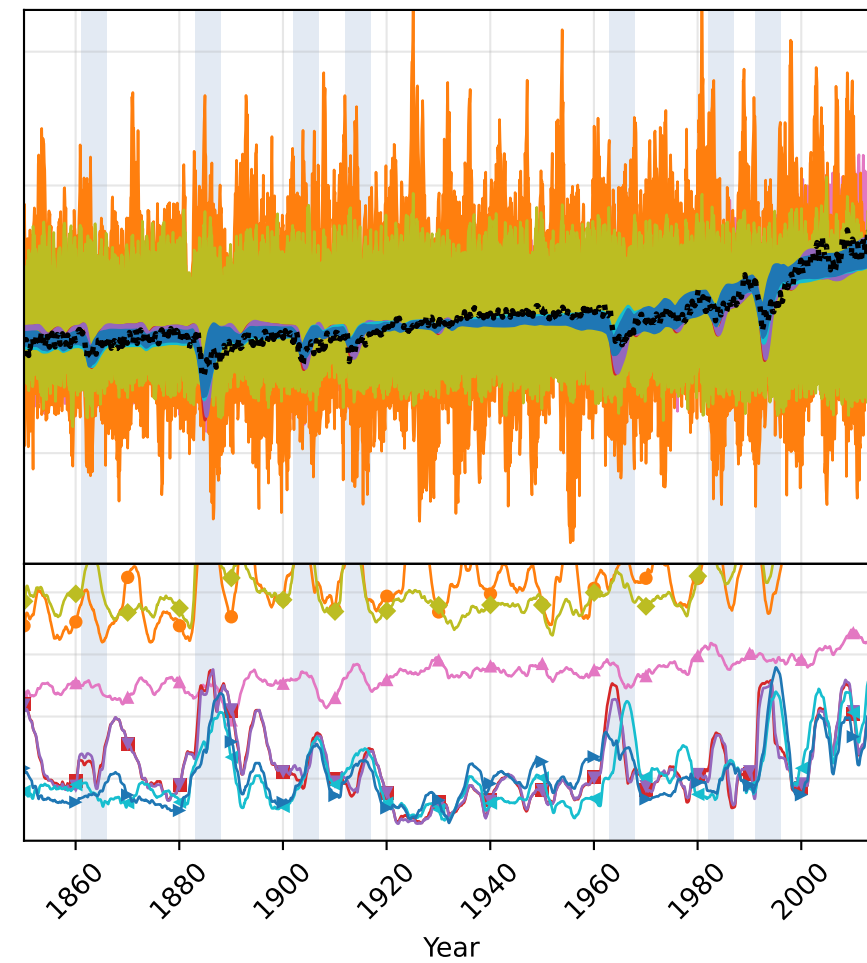
MIROC6
