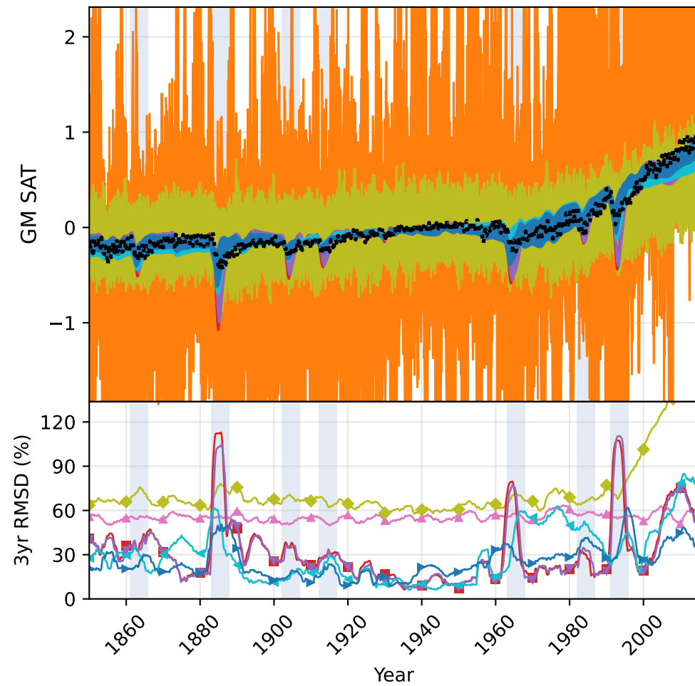
CESM2
