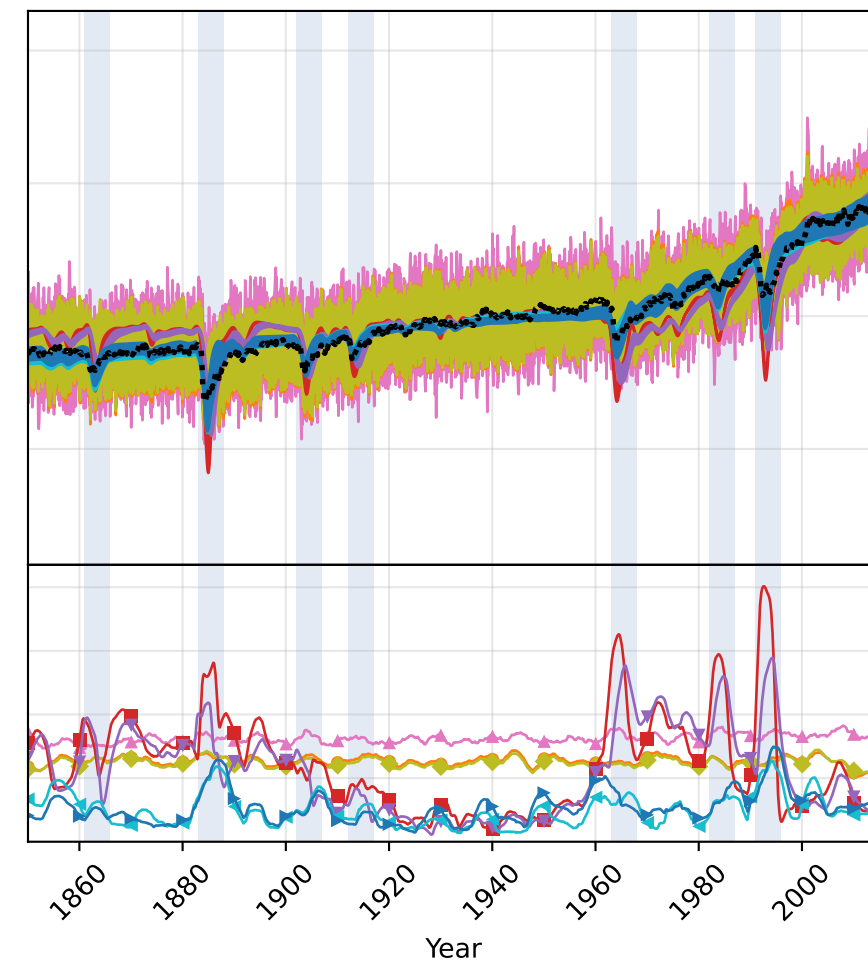
MPI-ESM
