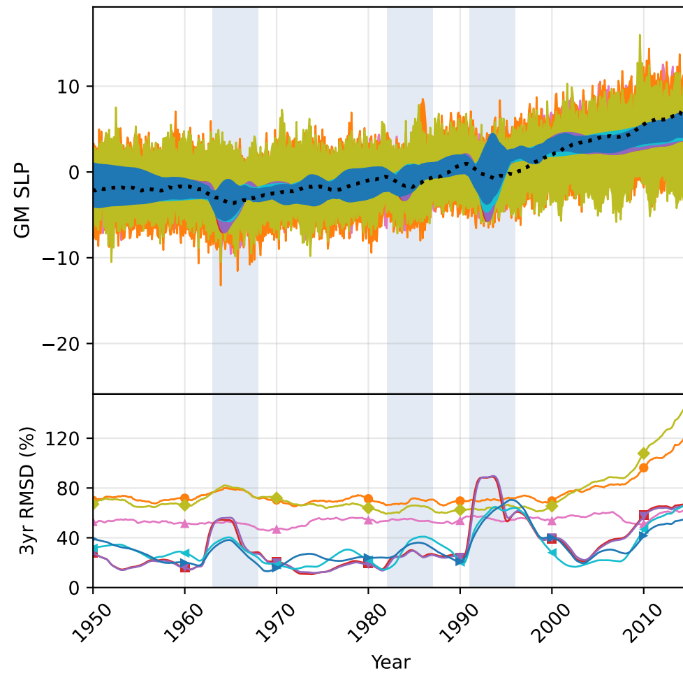
CESM2
