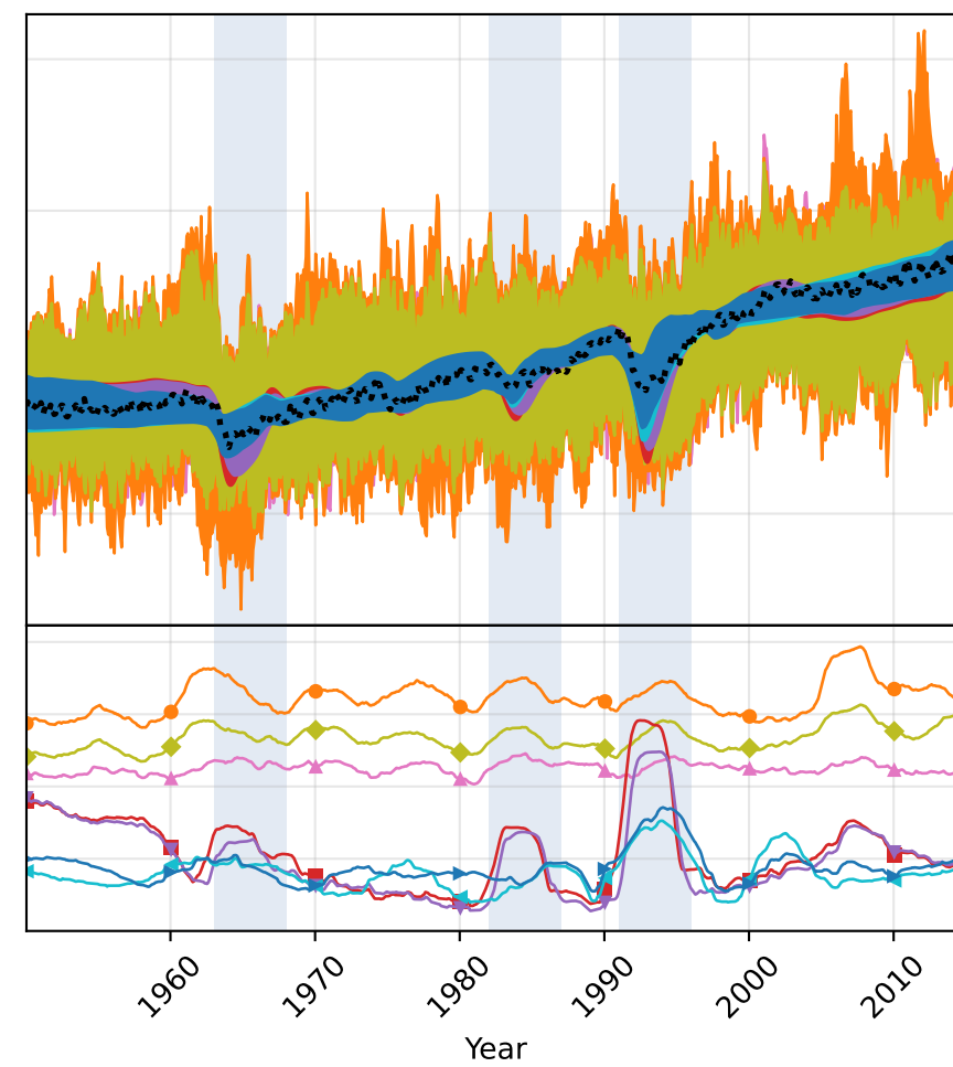
MPI-ESM
