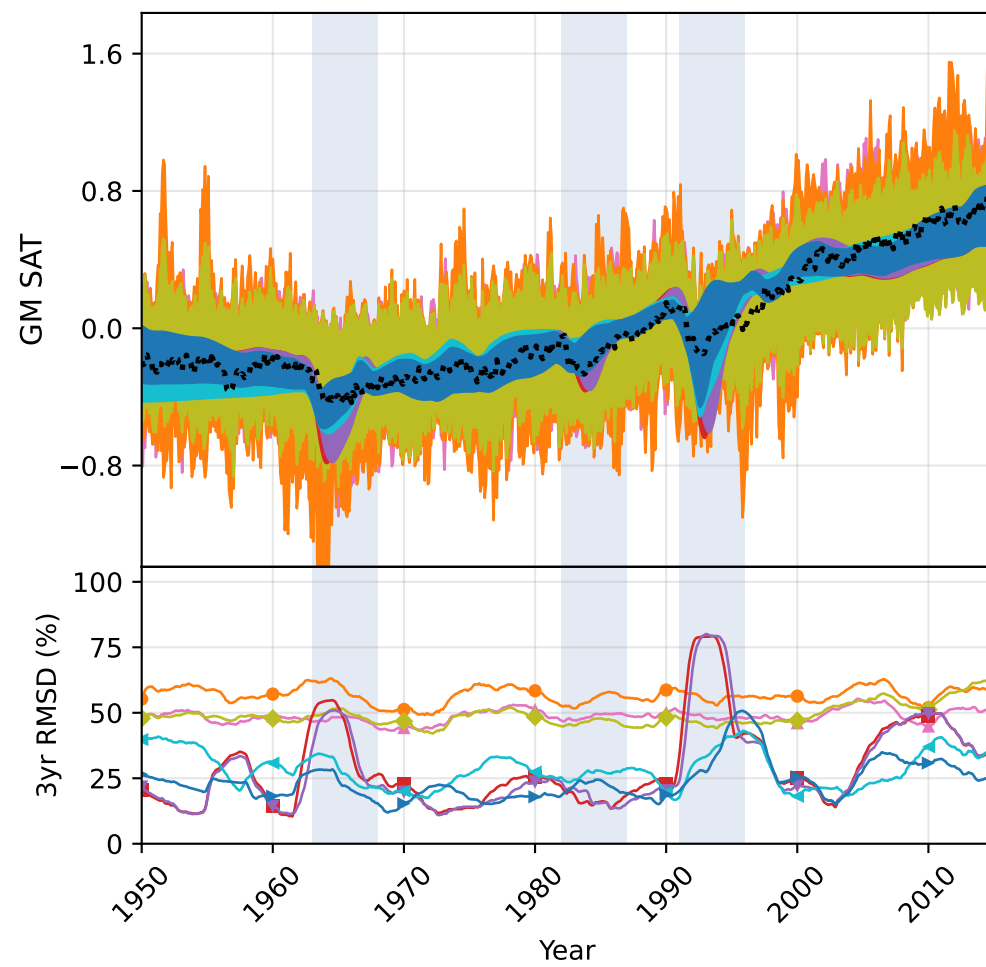
CESM2
