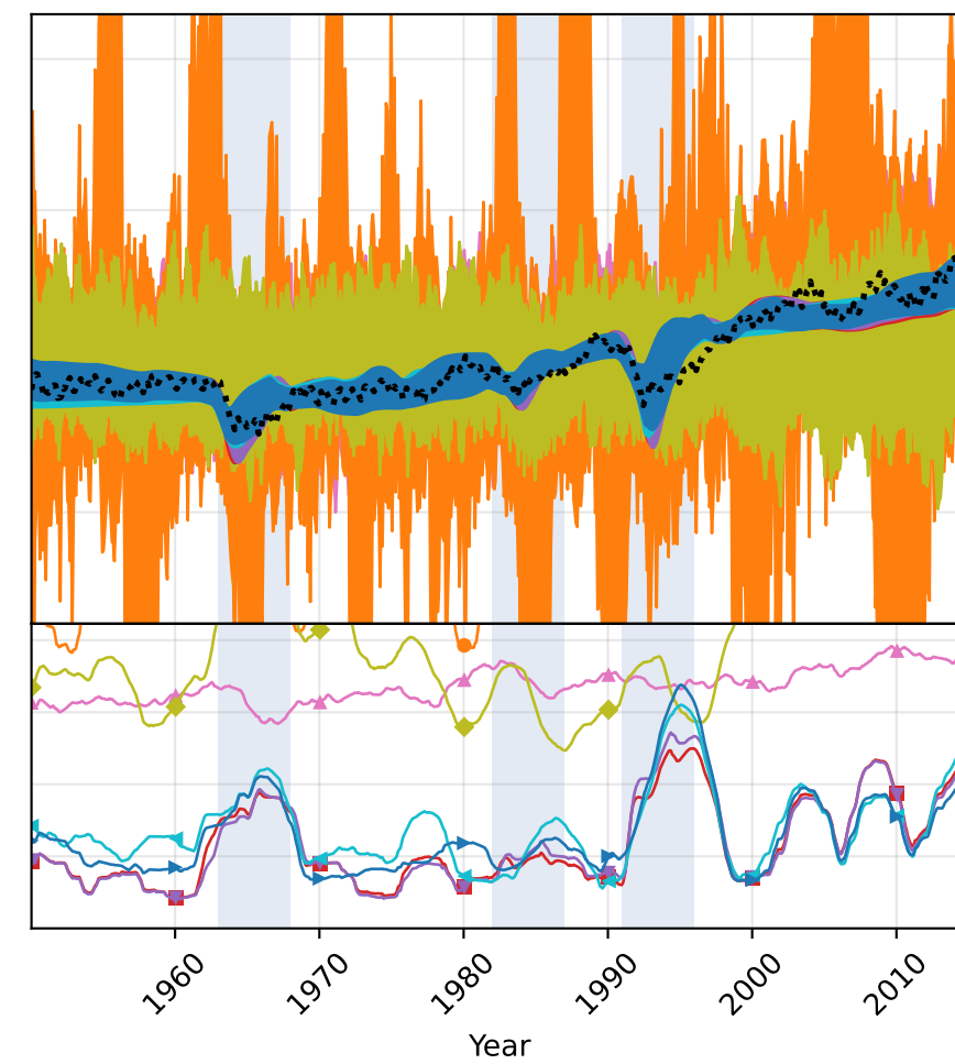
MIROC6
