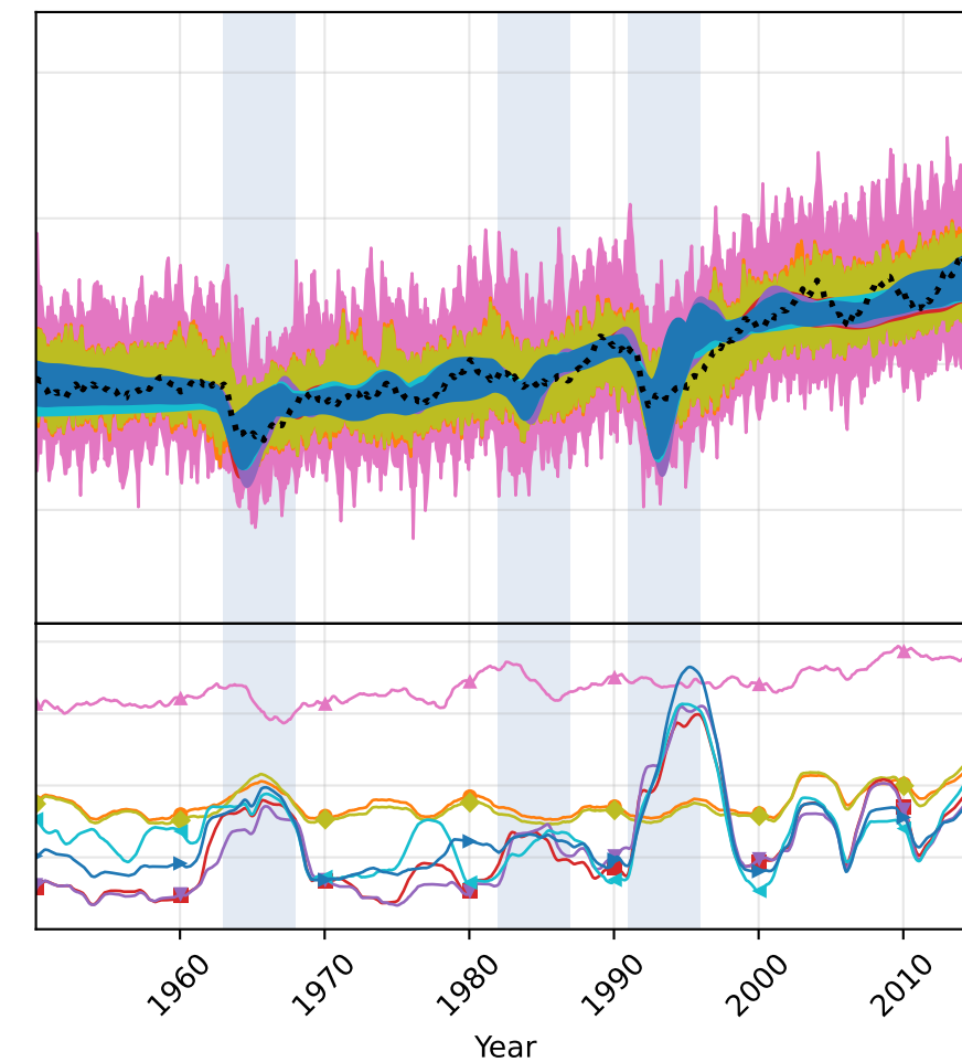
MIROC6
