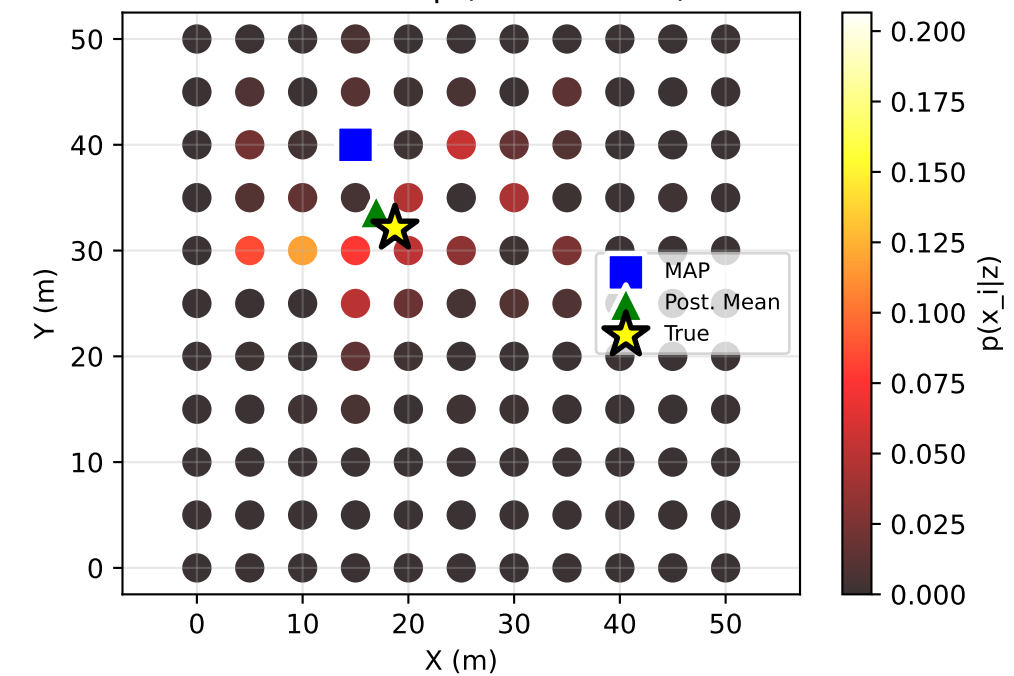
Posterior Map (std=5.0dBm)
