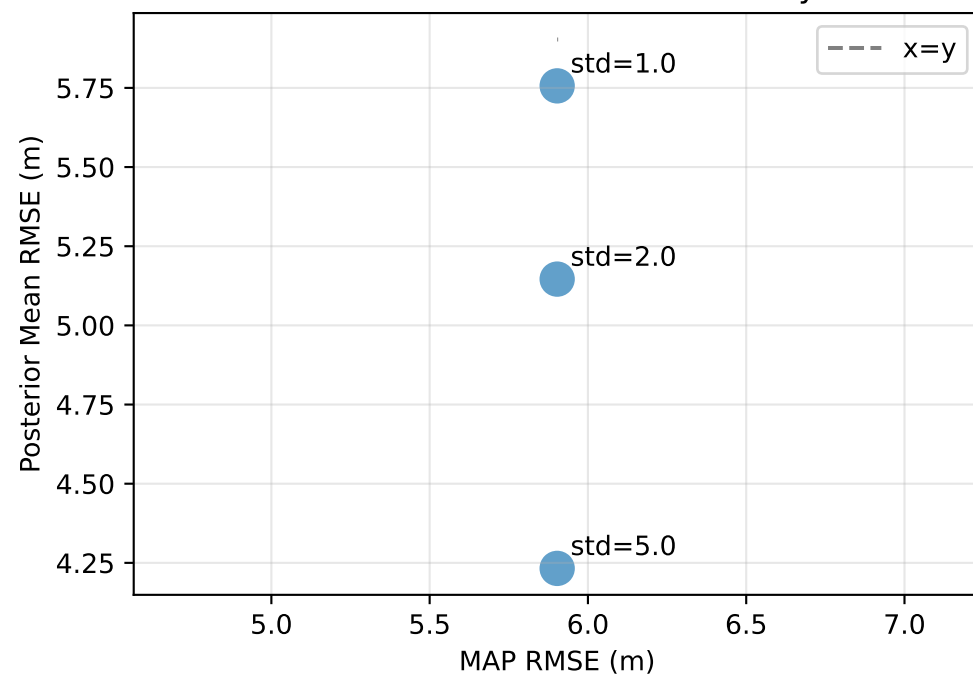
MAP vs Posterior Mean Accuracy
