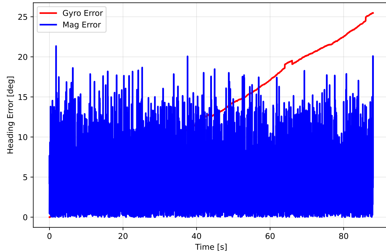
Heading Error
