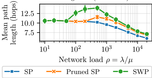
Cogentco (197 nodes)
