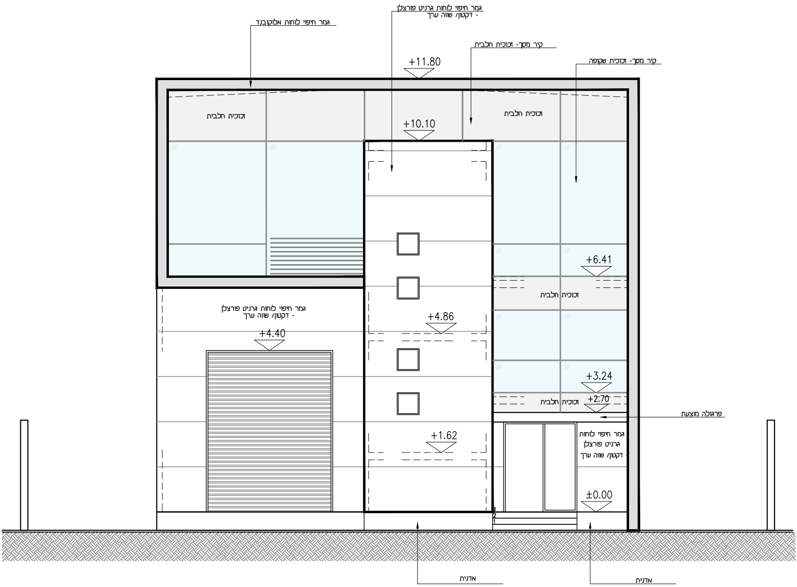
חזית דרומית קנ"מ 1:100
