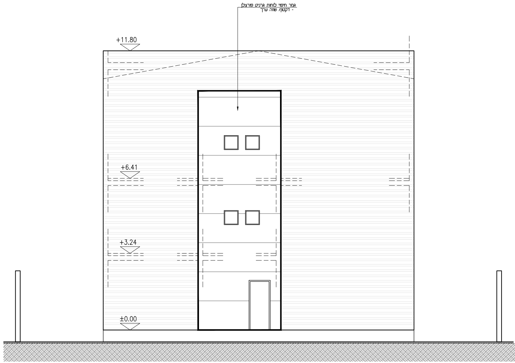
חזית צפונית קנ"מ 1:100
