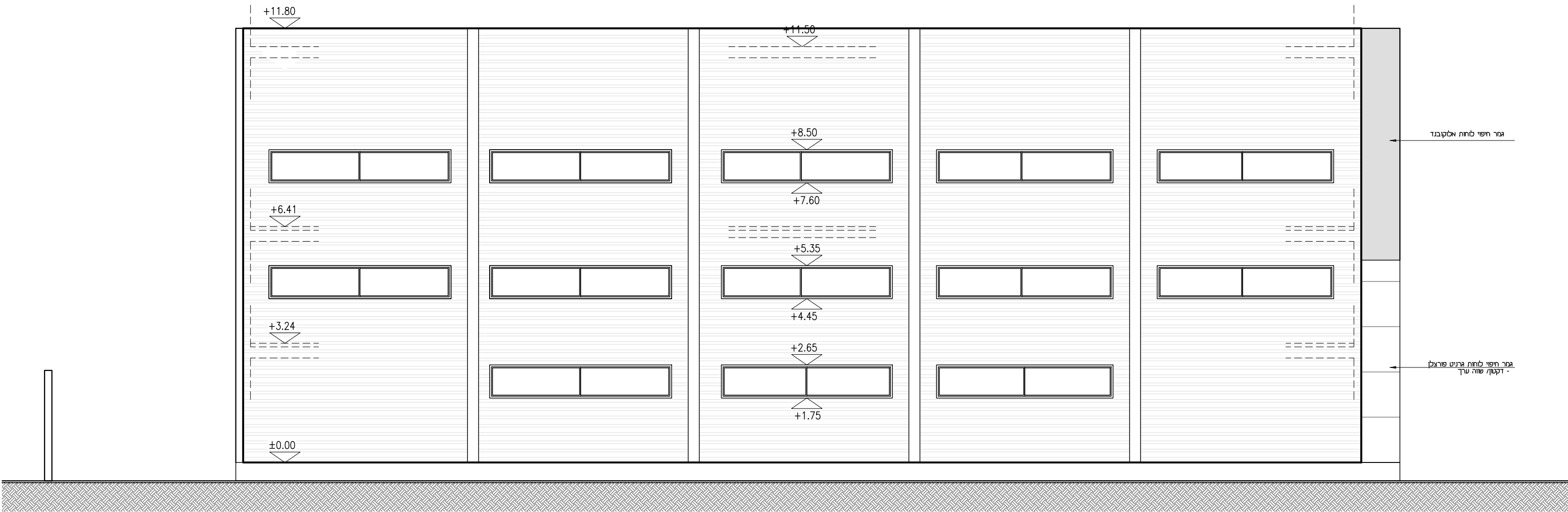
חזית מזרחית קנ"מ 1:100
