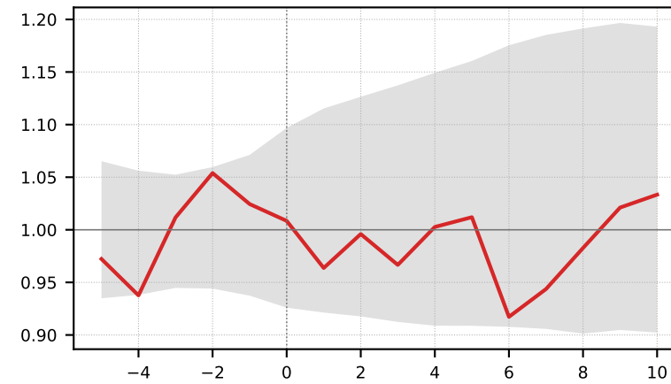
Moshiri (n=4, p=0.438)
