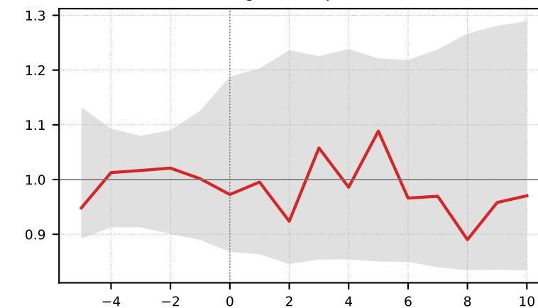
Omogo (n=6, p=0.364)
