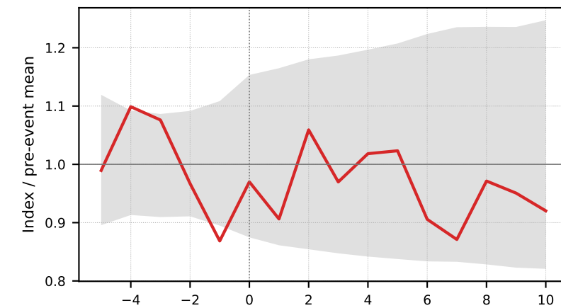
Onnebetsu (n=10, p=0.246)
