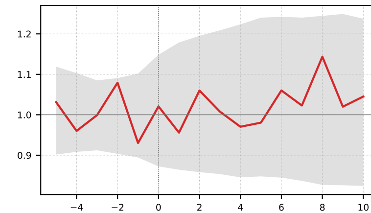
Senjo (n=8, p=0.569)
