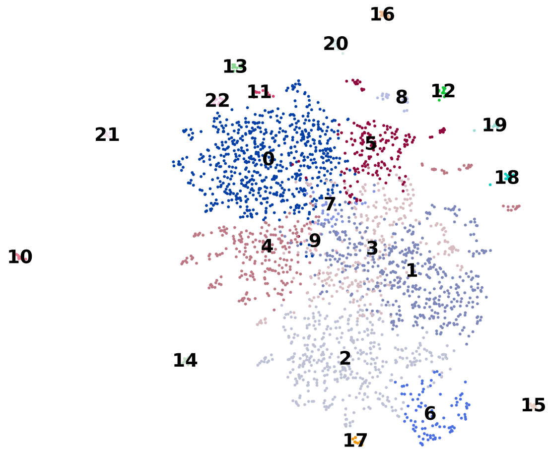
F_fre_rna (UMAP)
