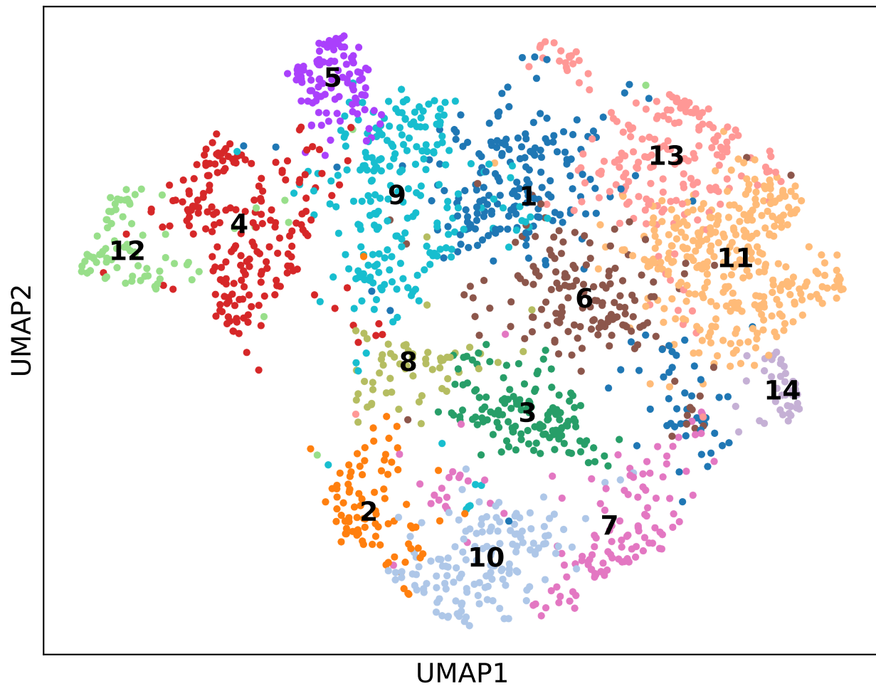
UMAP
