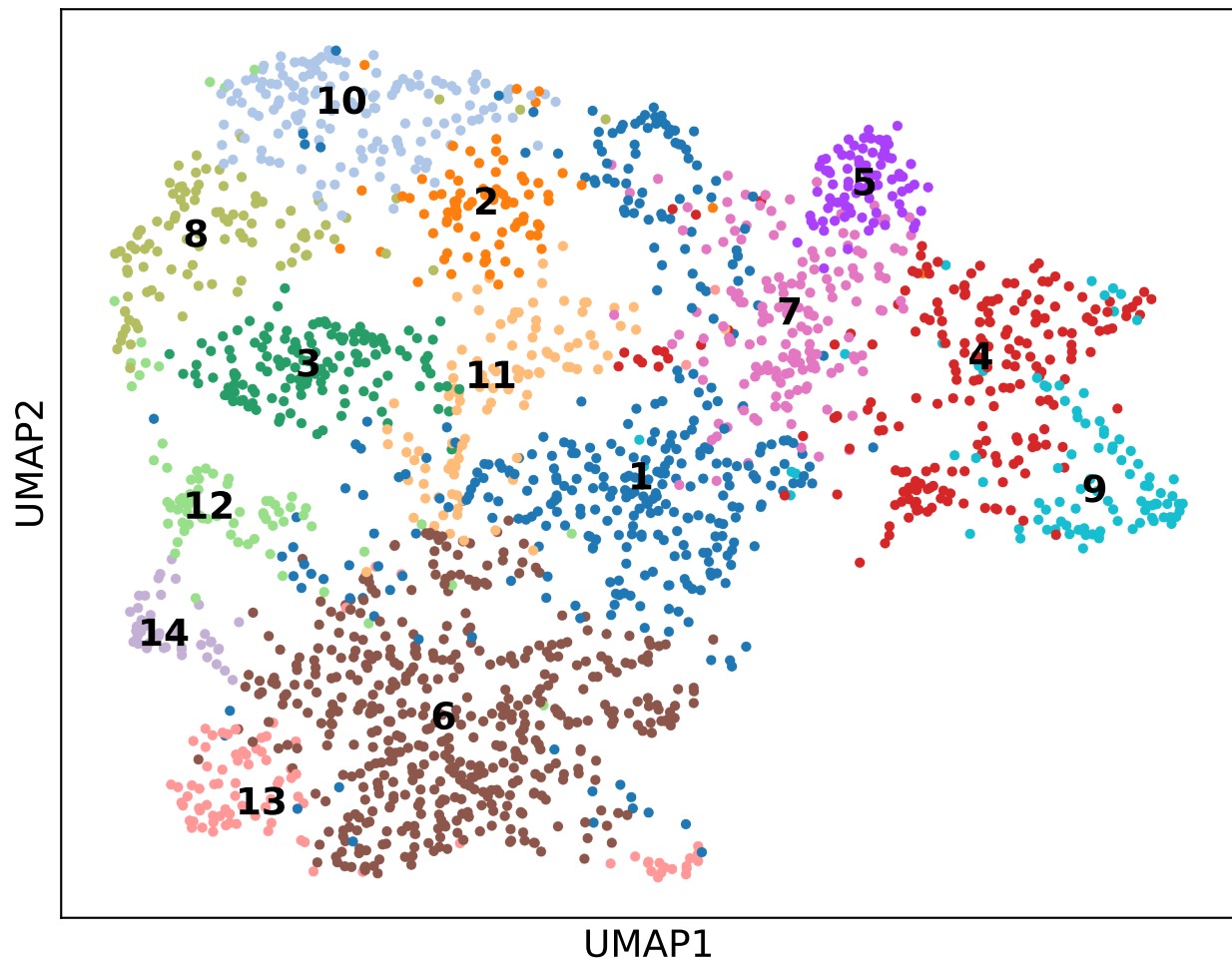
UMAP
