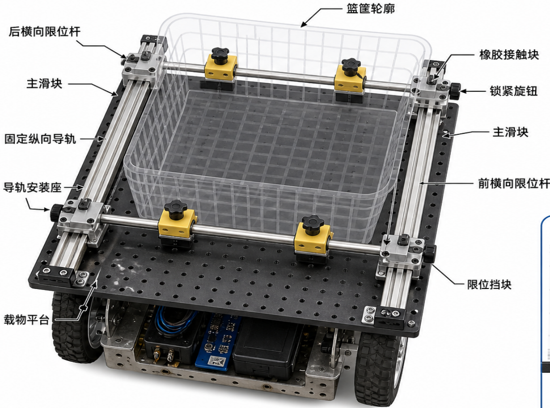
可调节的篮筐固定组件 – 组装示意图
