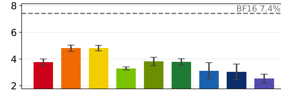
Gemma 3 12b
