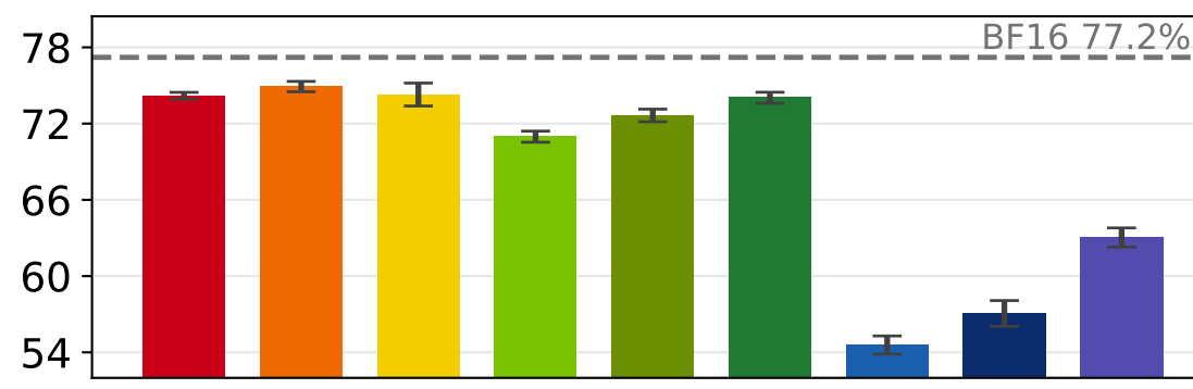
Gemma 3 12b
