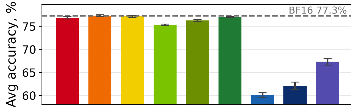
Gemma 3 4b
