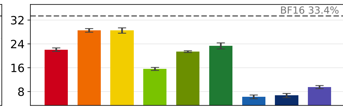
Gemma 3 1b
