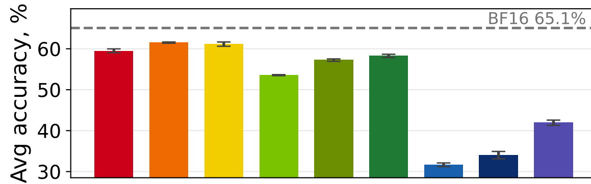
Gemma 3 4b
