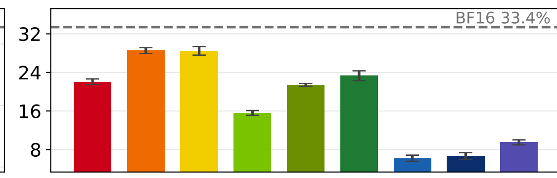
Gemma 3 1b
