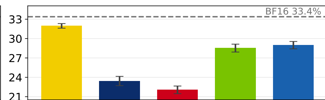
Gemma 3 1b
