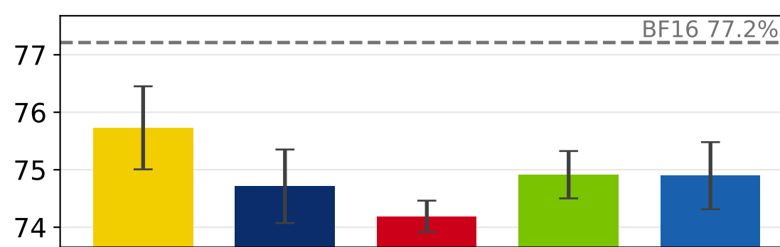
Gemma 3 12b
