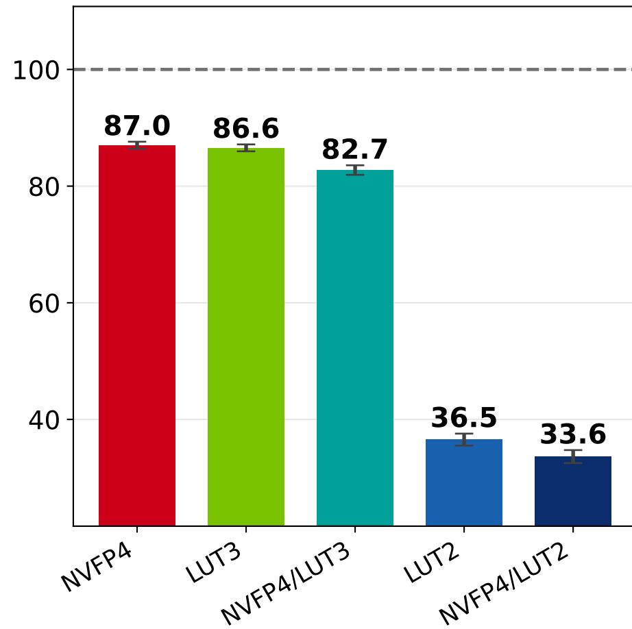
Qwen3-1.7B
