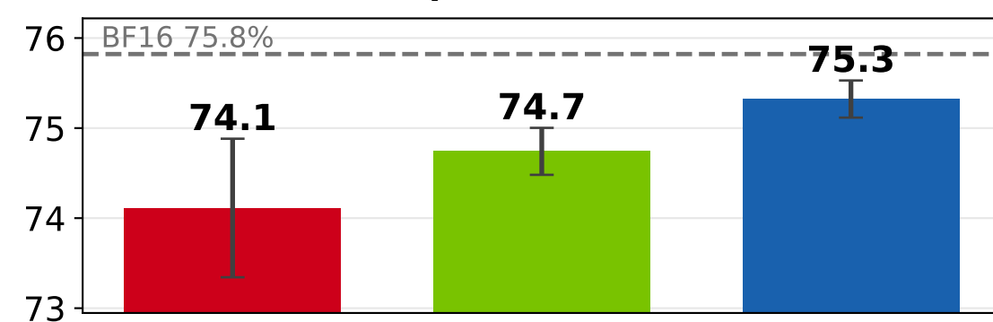
Gemma 3 1b
