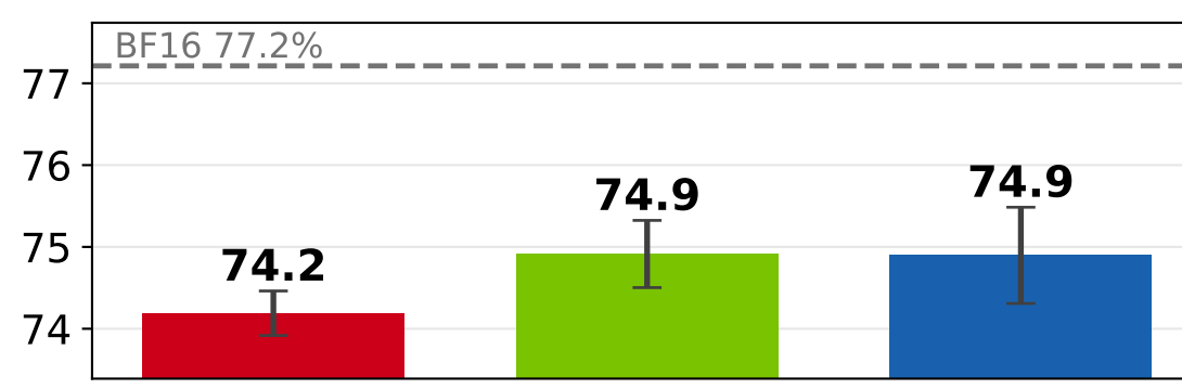
Gemma 3 12b
