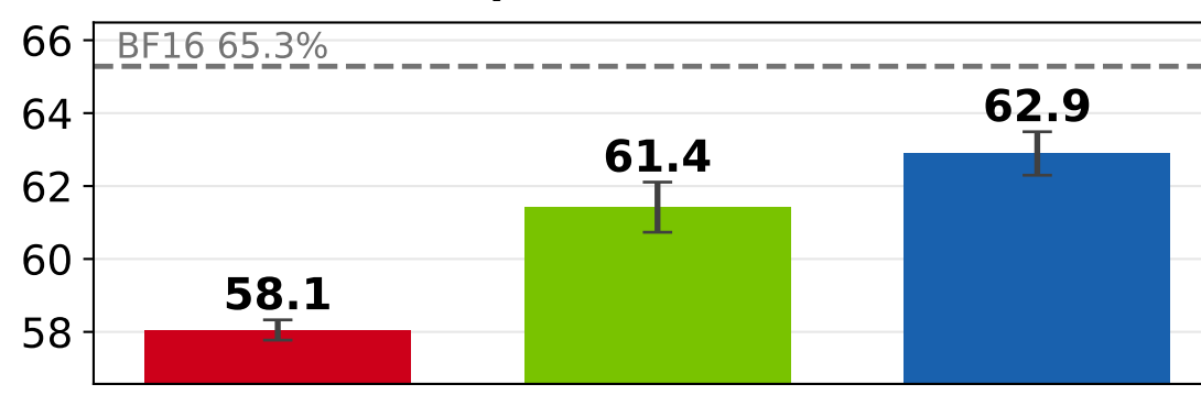
Gemma 3 270m
