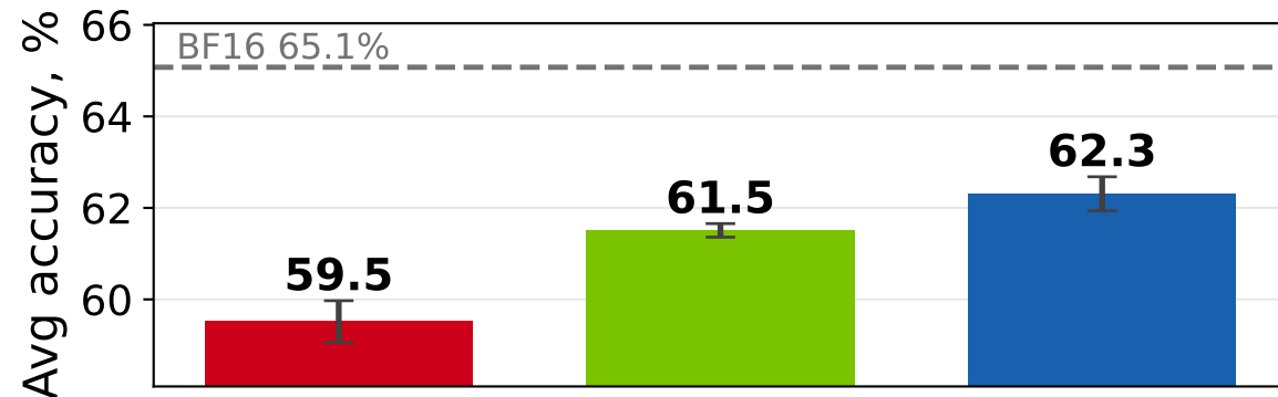
Gemma 3 4b
