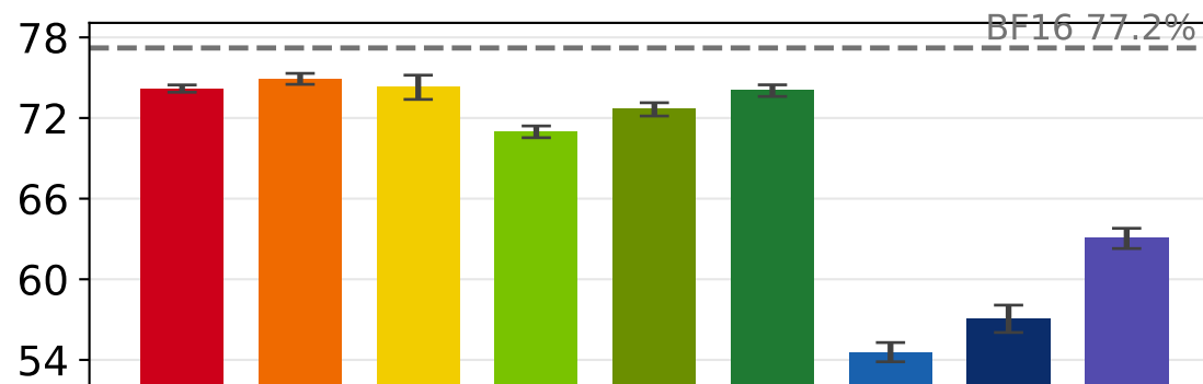
Gemma 3 12b
