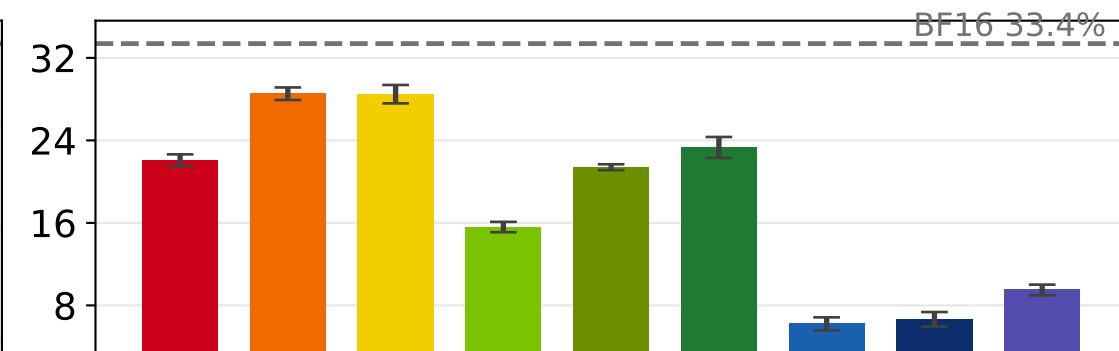
Gemma 3 1b
