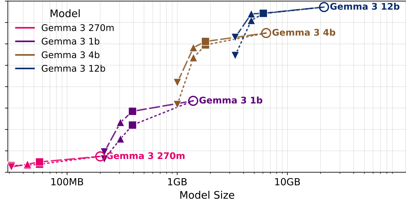
Gemma 3
