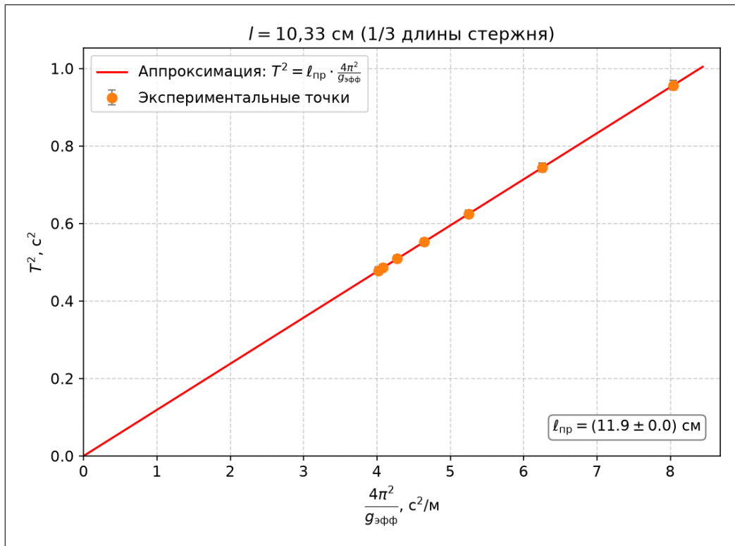
Рис. 4: Зависимость T^2 от 4\pi^2/g_{\text{эфф}} для l = 10.33 \text{ см}
