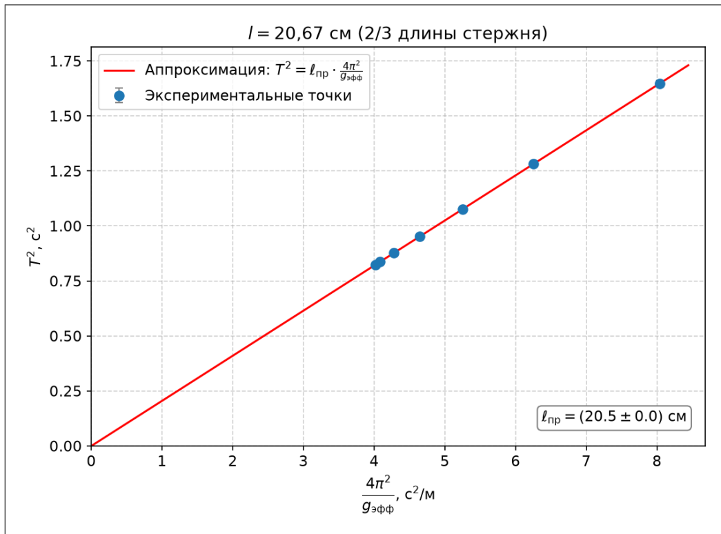
Рис. 2: Зависимость T^2 от 4\pi^2/g_{\text{эфф}} для l = 20.67 \text{ см}
