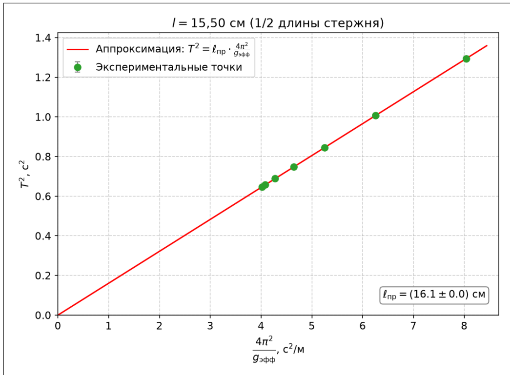
Рис. 3: Зависимость T^2 от 4\pi^2/g_{\text{эфф}} для l = 15.50 \text{ см}
