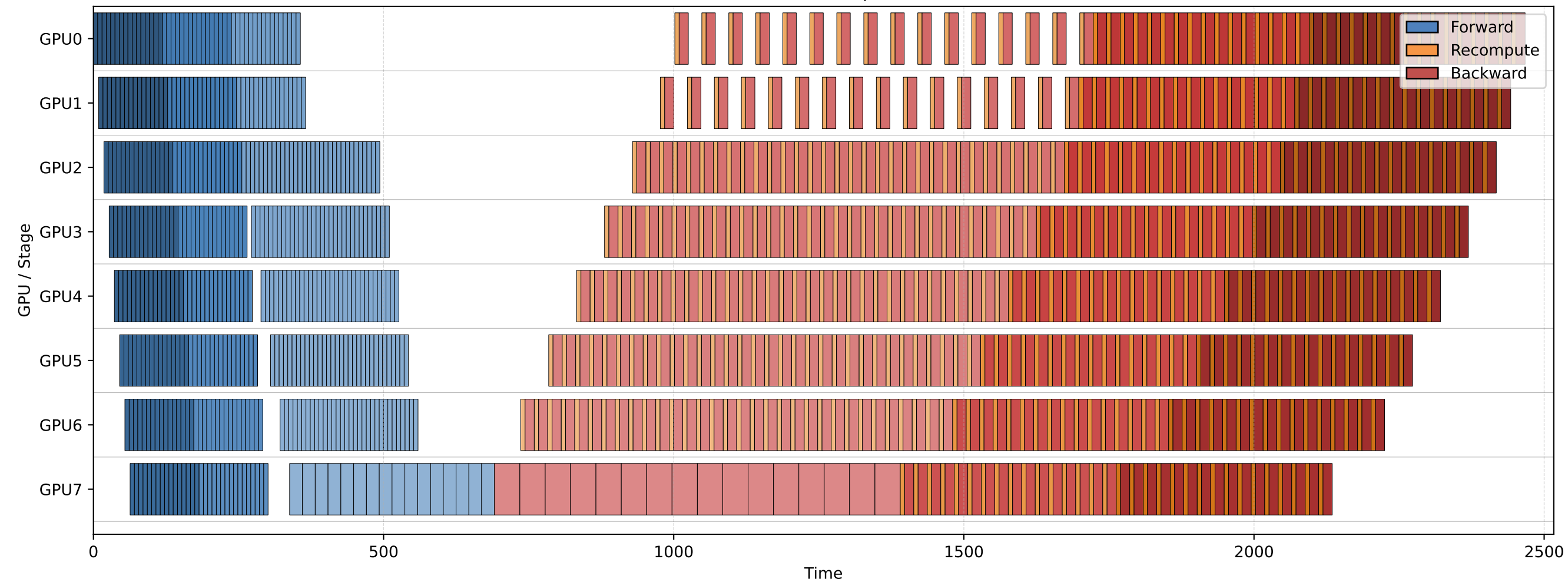
Qwen3-1.7B Looped-BFS
