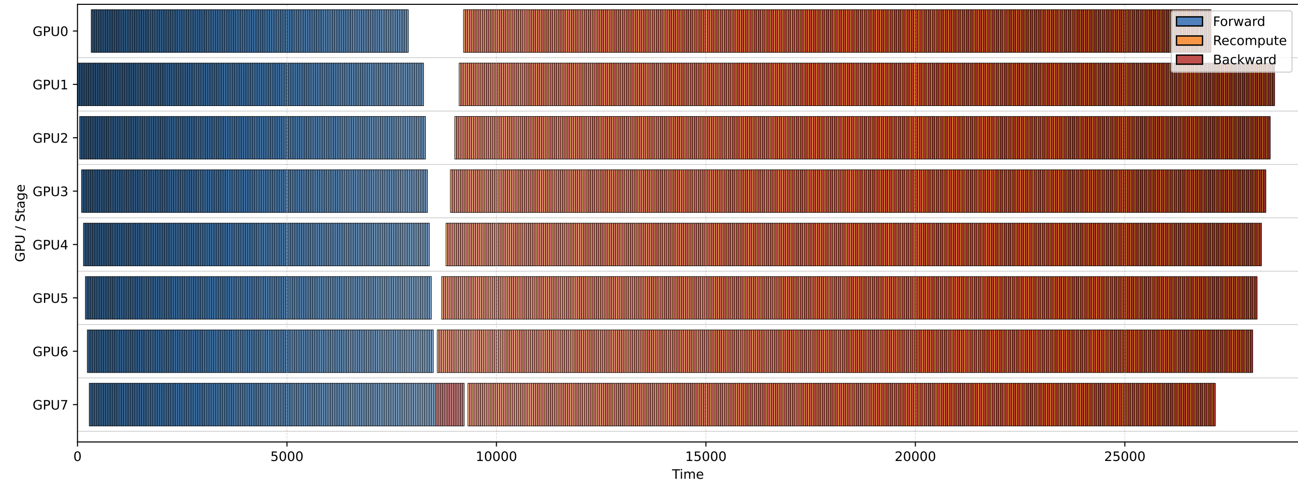
Qwen3-235B Looped-BFS
