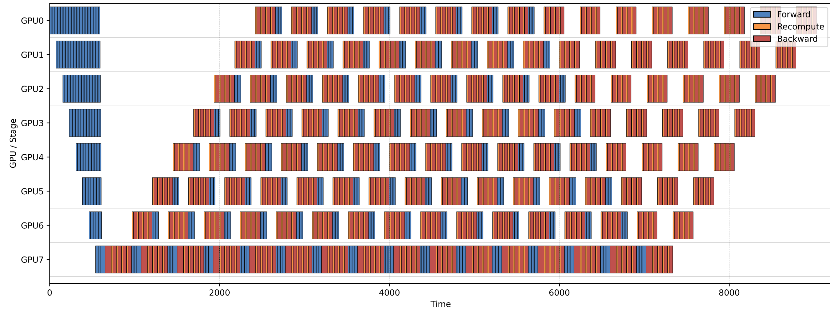
Llama3-8B 1F1B
