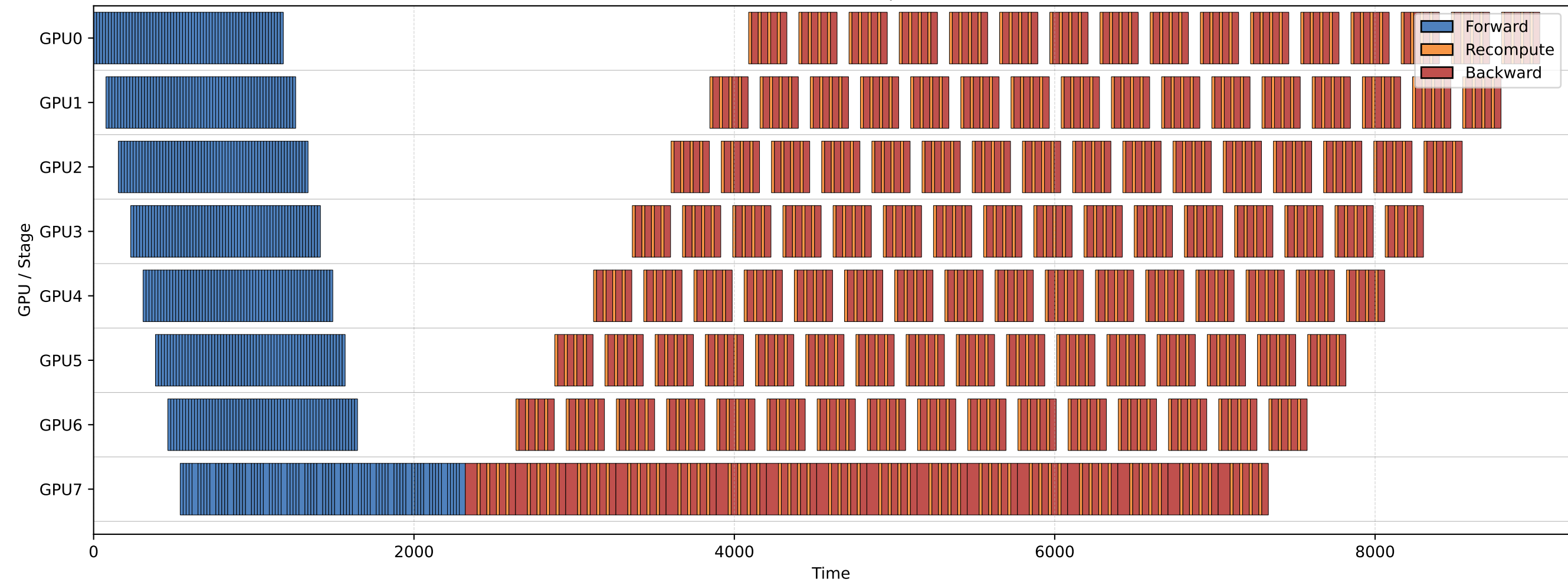
Llama3-8B GPipe
