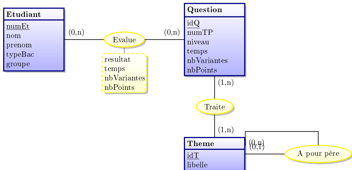
Figure 2 – Modèle conceptuel des données (MCD)
