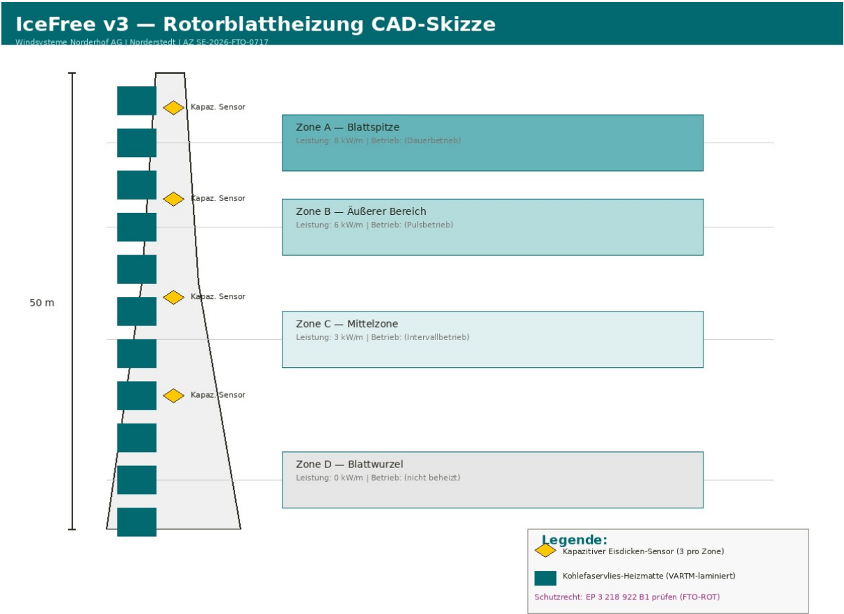
Bilddatei: rotorblattheizung-cad-zeichnung.jpg
