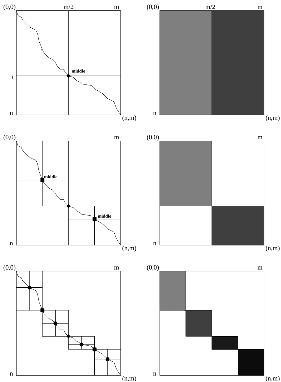
Figura 3.1: Suddivisione ricorsiva dello spazio di allineamento nell'algoritmo in spazio lineare. Tratto da Jones e Pevzner [JP04, p. 235].
