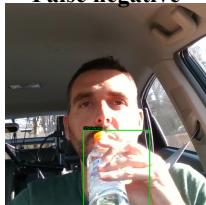
YOLO26n
