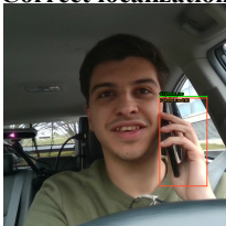
YOLO26n
