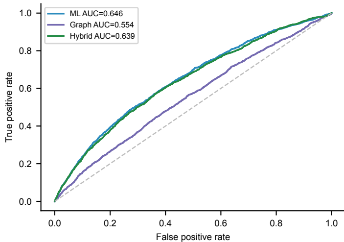
ROC
