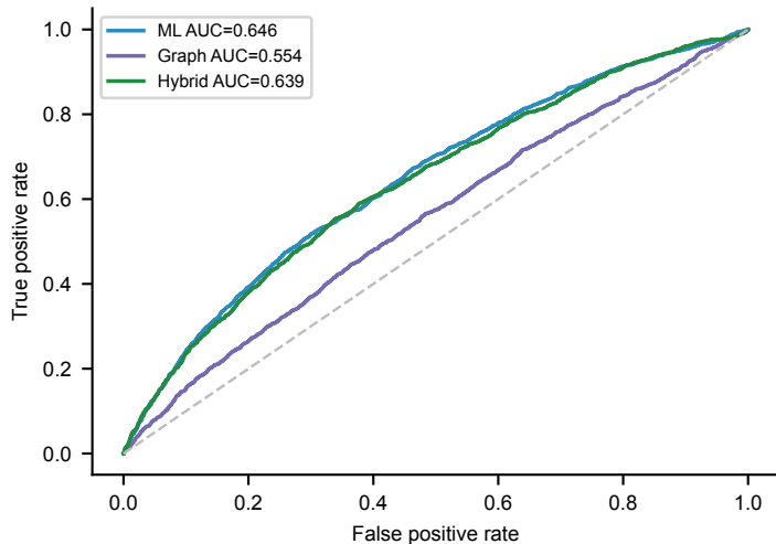
ROC
