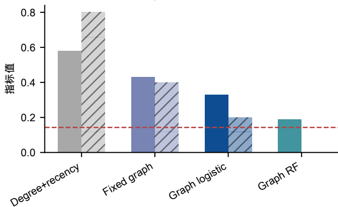
b 时间留出 2025
