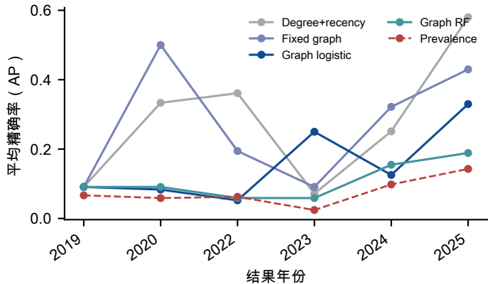
a 逐年前向回测
