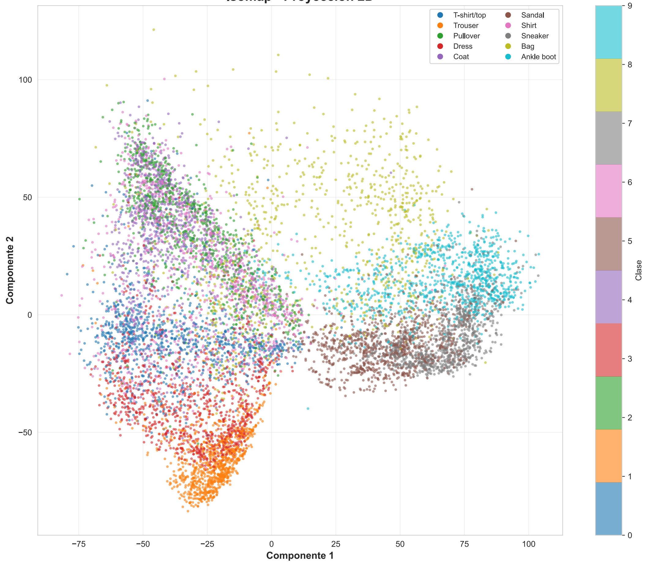
Isomap - Proyección 2D
