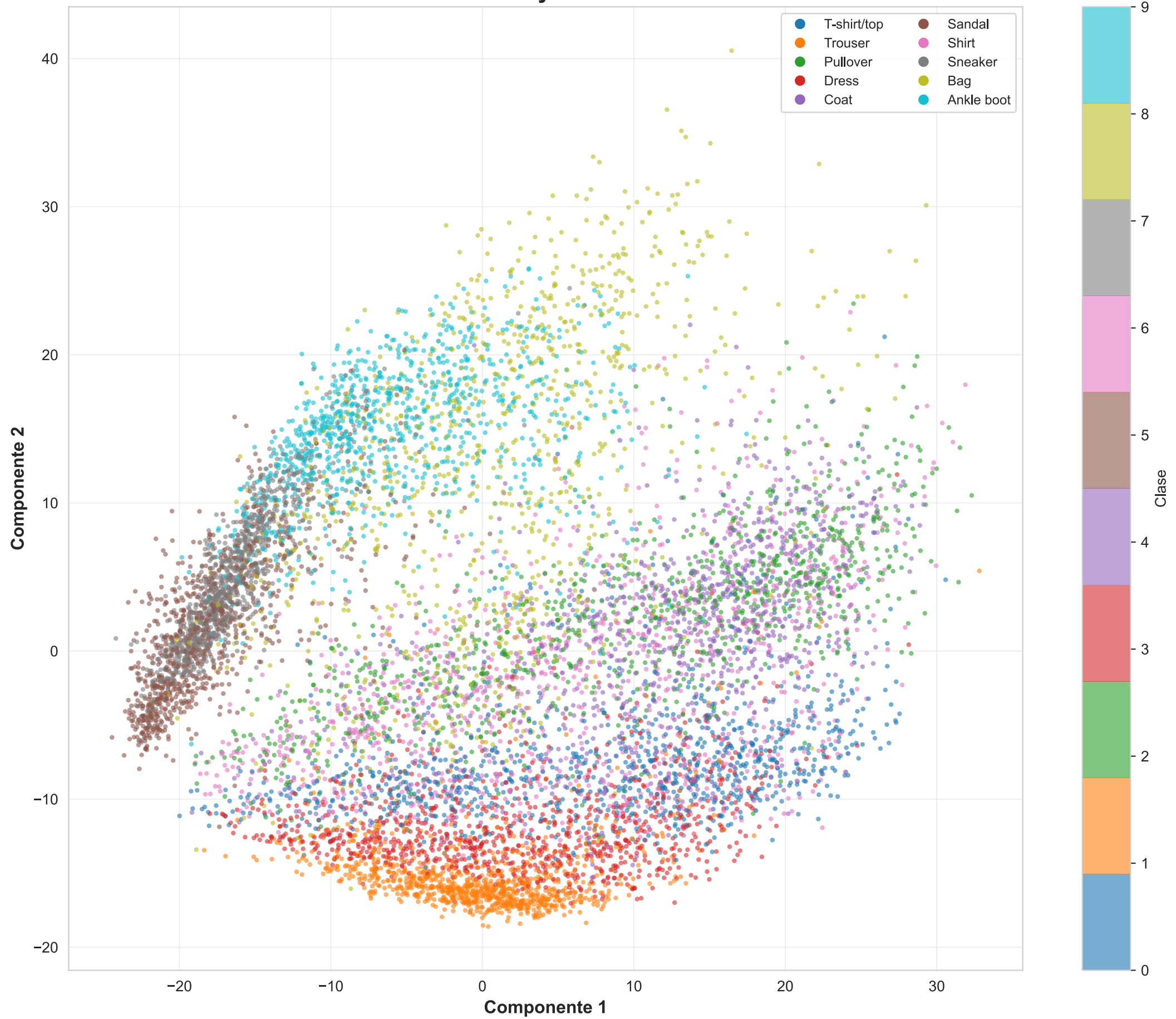
PCA - Proyección 2D
