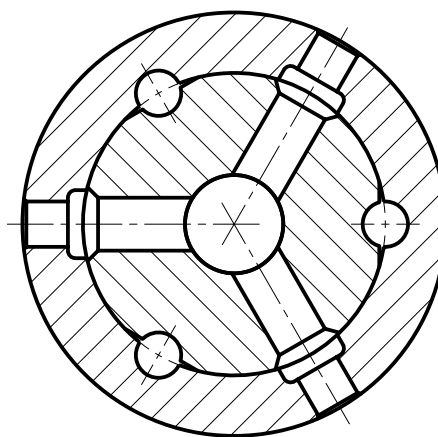
Д-Д (1:1)
