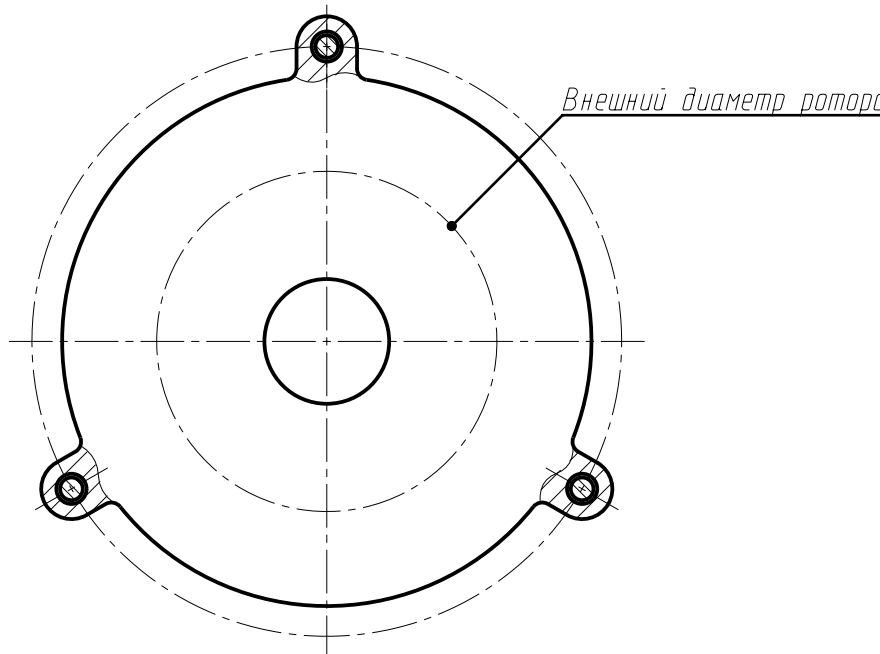
И-И (1:2)
