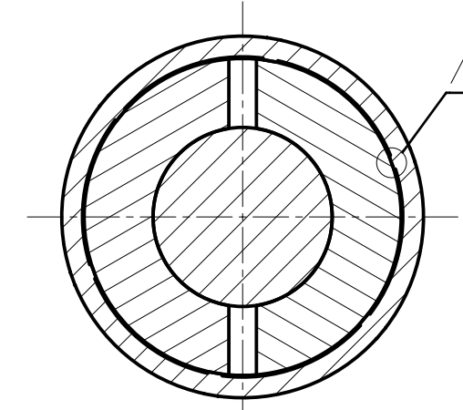
Е-Е (1:1)
