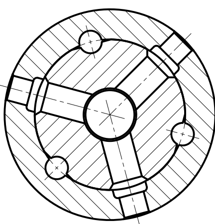
Г-Г (1:1)
