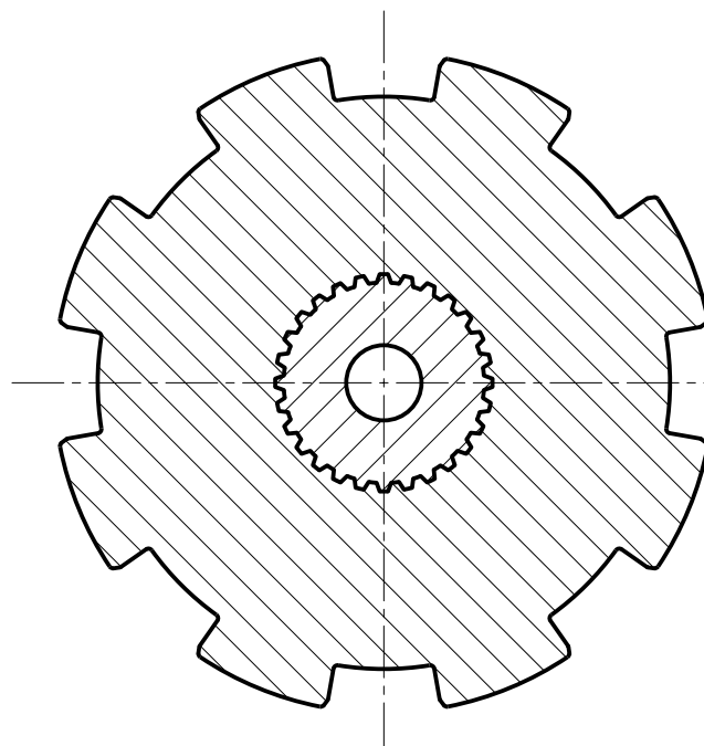
Ж-Ж (1:1)
