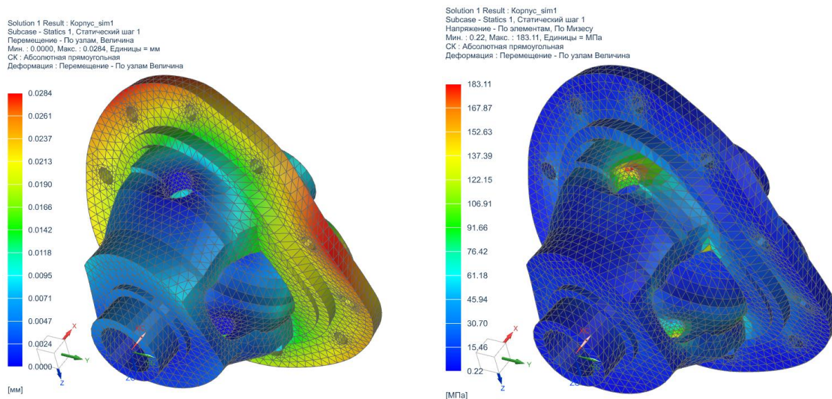
Рисунок 26 – Эпюры деформаций (слева) и напряжений (справа)
