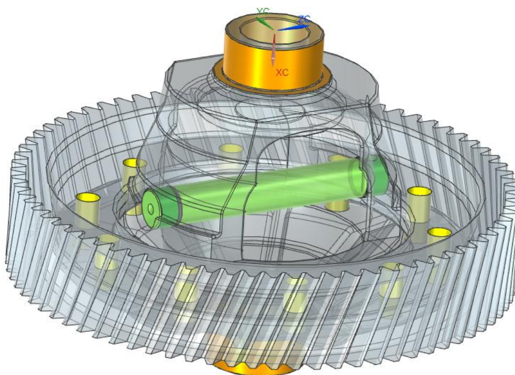
Рисунок 48 – Сборка дифференциала
