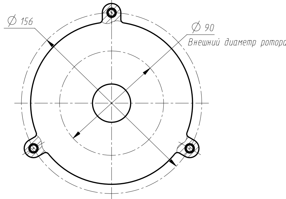
И-И (1:2)
