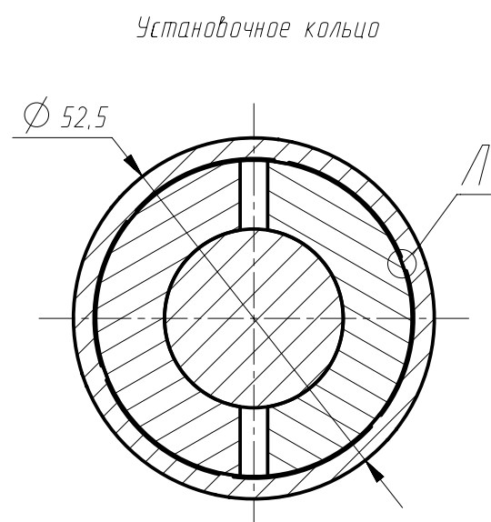
Е-Е (1:1)
