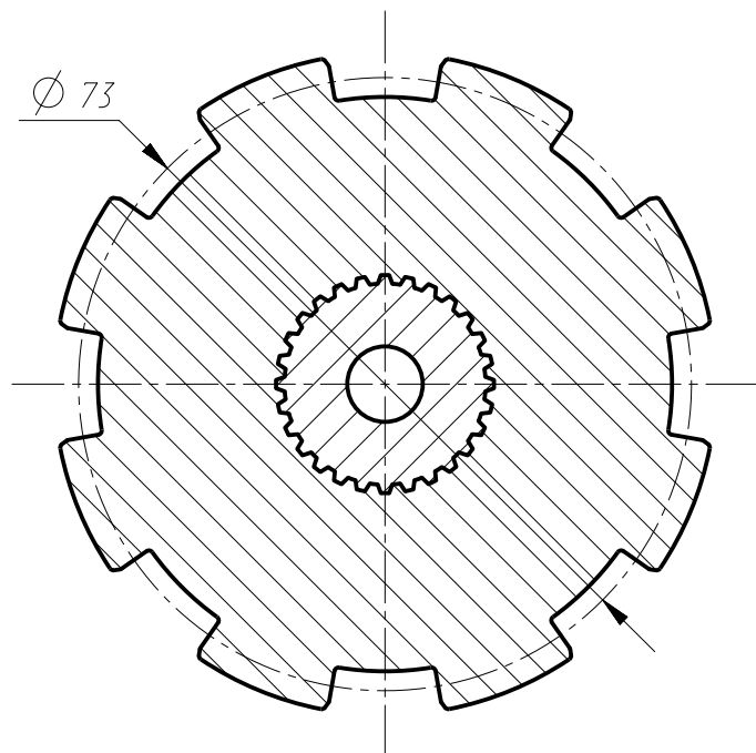
Ж-Ж (1:1)
