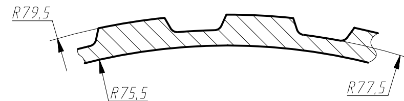
Б-Б (1:1) Редра жесткости
