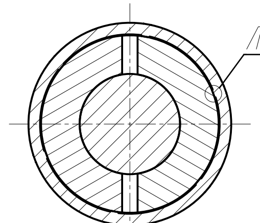
Е-Е (1:1) Установочное кольцо
