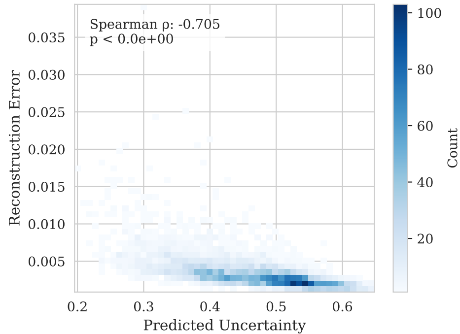
Vanilla VAE
