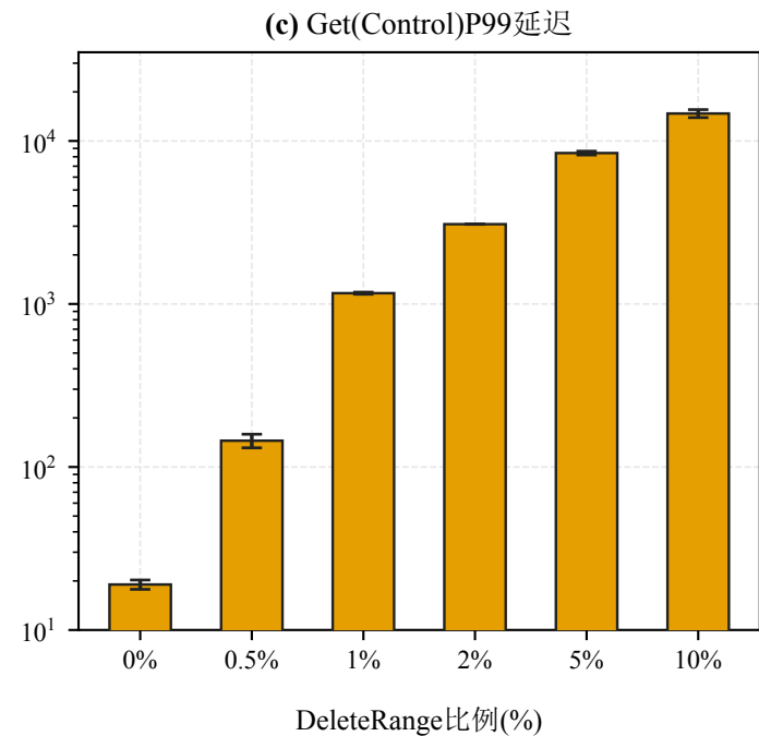
Get(Control)P99( \mu s, 对数坐标)
