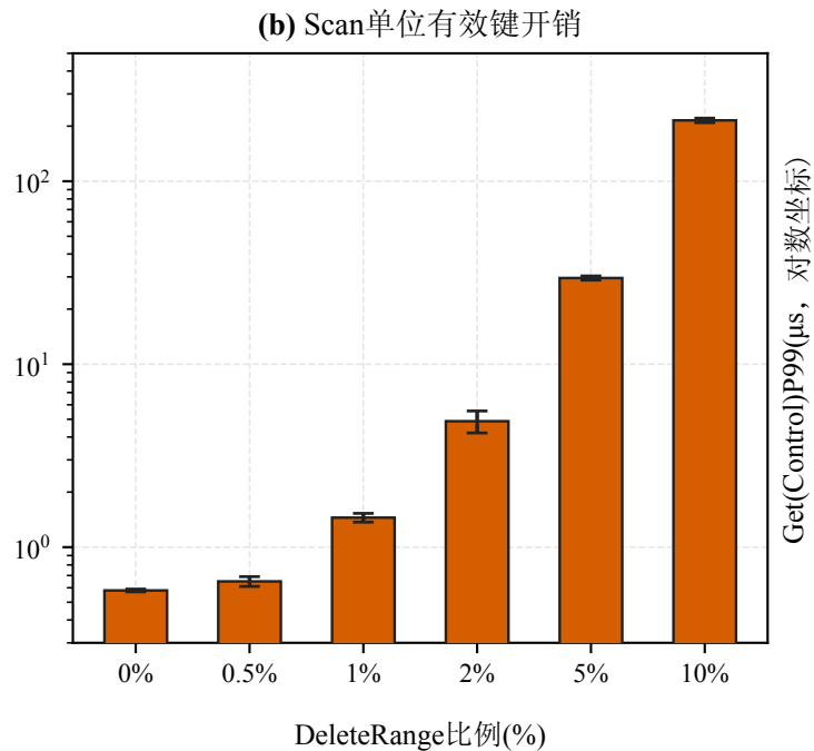
Scan开销( \mu s/key, 对数坐标)
