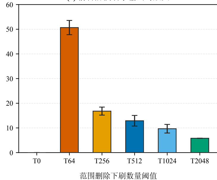
(c) 前台阶段引擎输出写放大
