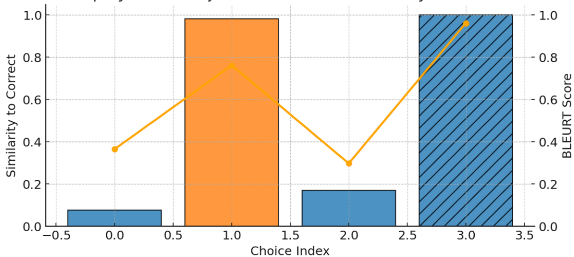
DisplayUserCard.json - Per-choice Similarity & BLEURT
