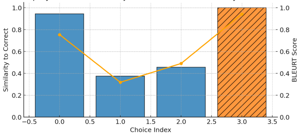
DisplayReservationCard.json - Per-choice Similarity & BLEURT
