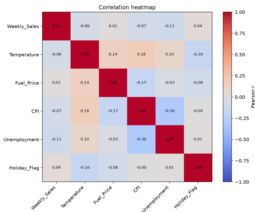
图 1: 主要变量间的 Pearson 相关热力图
