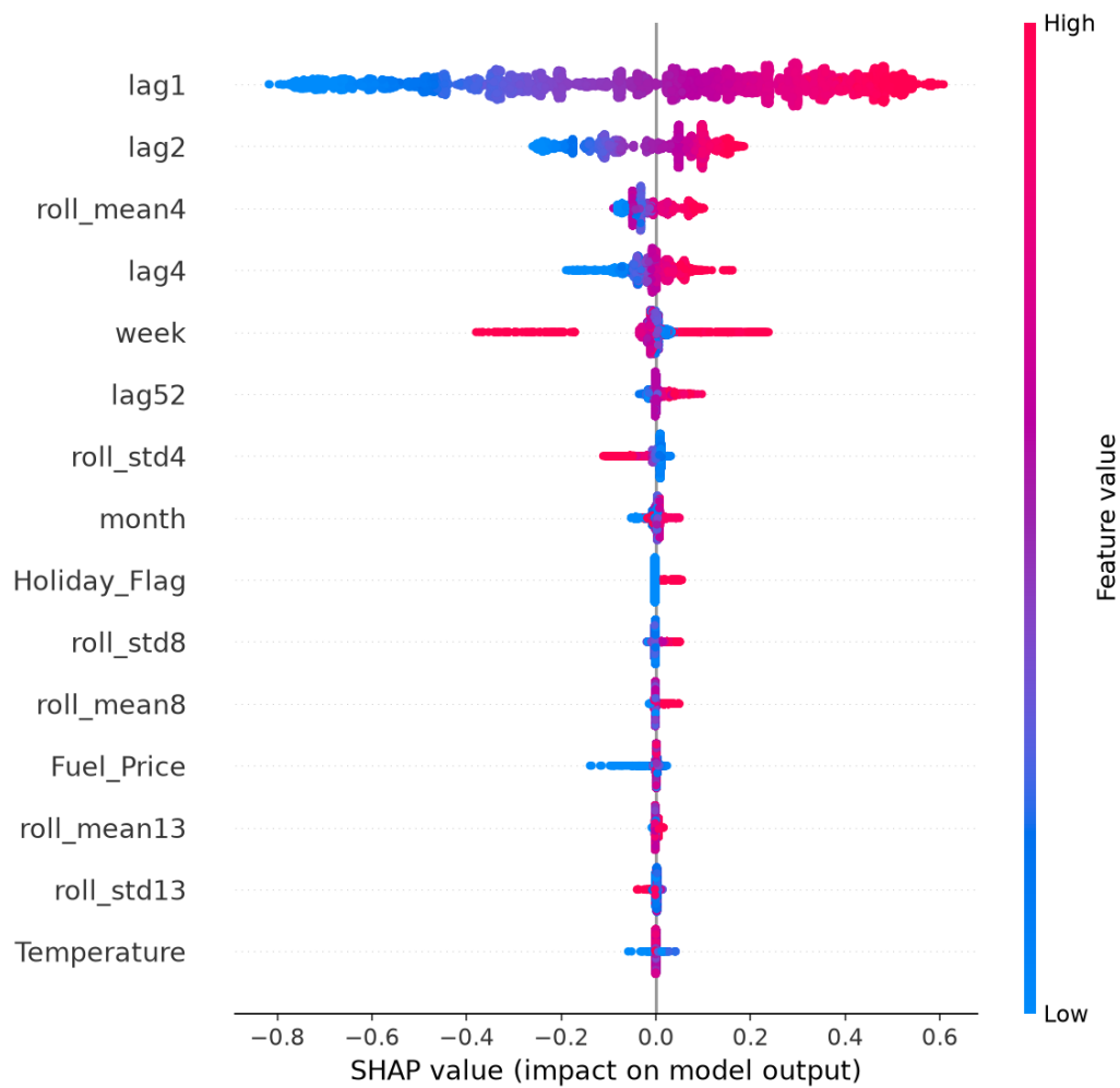
图 6: XGBoost 特征 SHAP 蜂群图 (特征集与最优模型一致, 不含门店哑变量)
