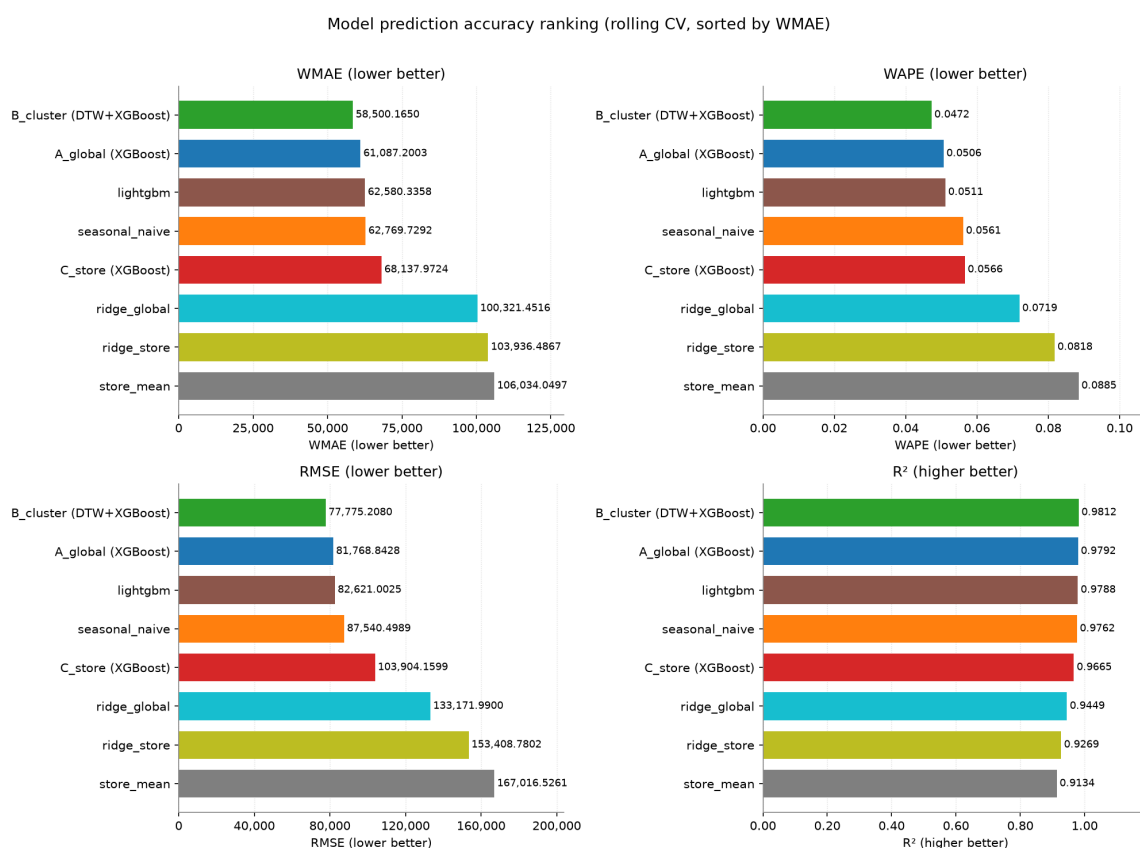
图 3: 模型预测准确率排名（横向柱状图，按 WMAE 排序）
