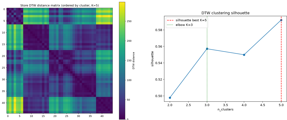
图 2：左：按簇排序的门店 DTW 距离矩阵；右：轮廓系数随簇数的变化（最优 K = 5 ）
