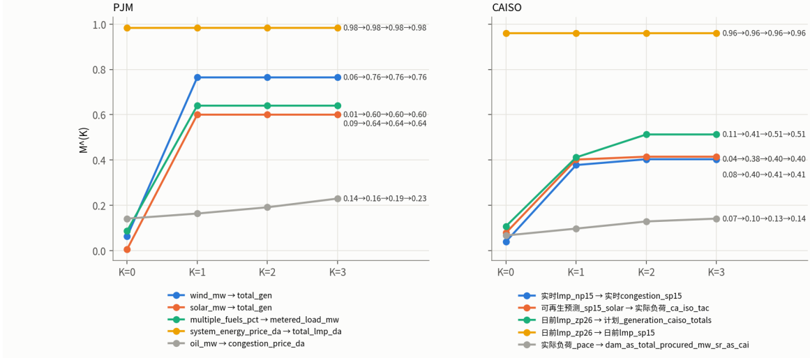
图2 典型推断升级曲线：单字段弱、一个辅助字段即跃升（出力+占比、节点价差），与单字段即强的字段对照
